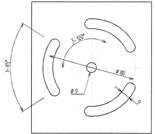
A 矢視 (底面図)
